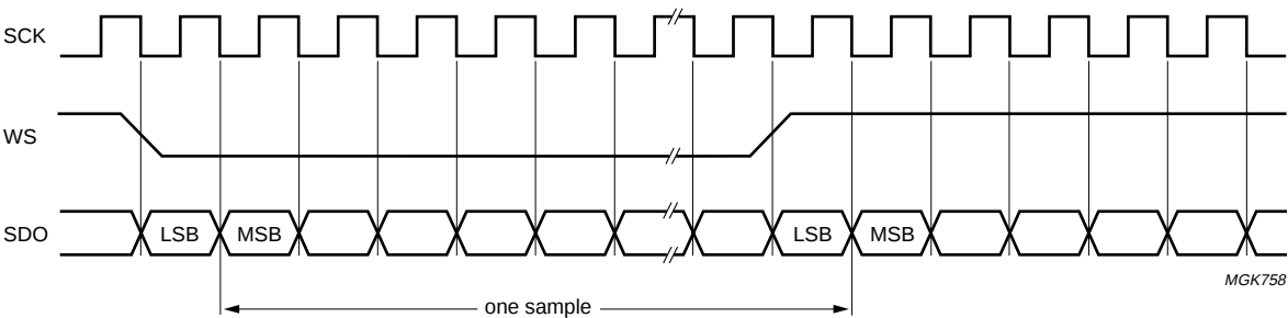
a. I²S-bus format.
